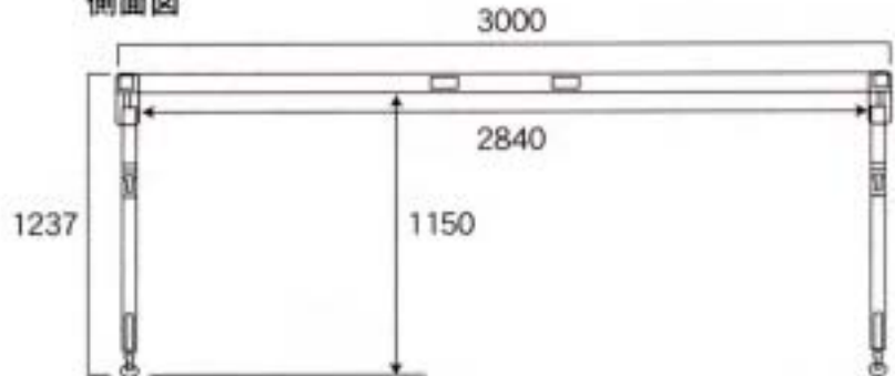
側面図
